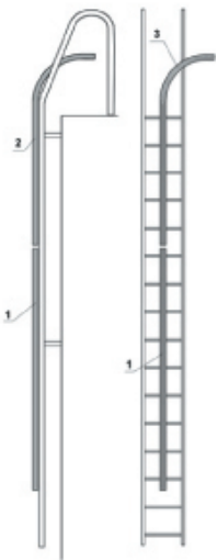
Turvavaruste 1: nousuturvakisko
